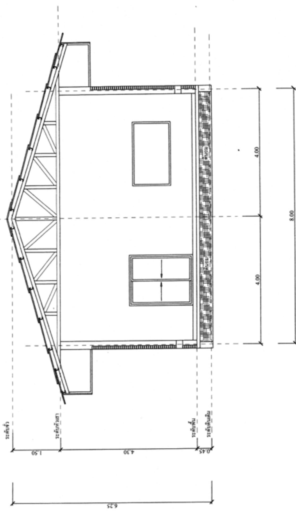
รูปตัดดัดใหม่ Scale 1:50
